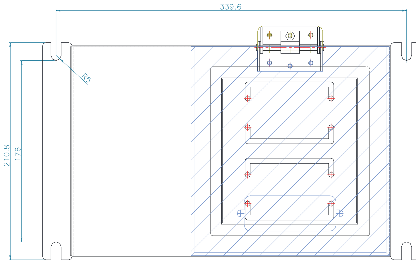
F2C 上から見た底面取り付け板の寸法図 (レールへのネジ止め部)
